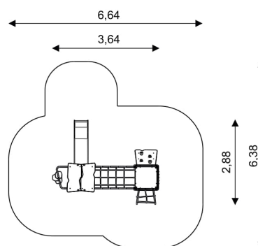
Przestrzeń minimalna
